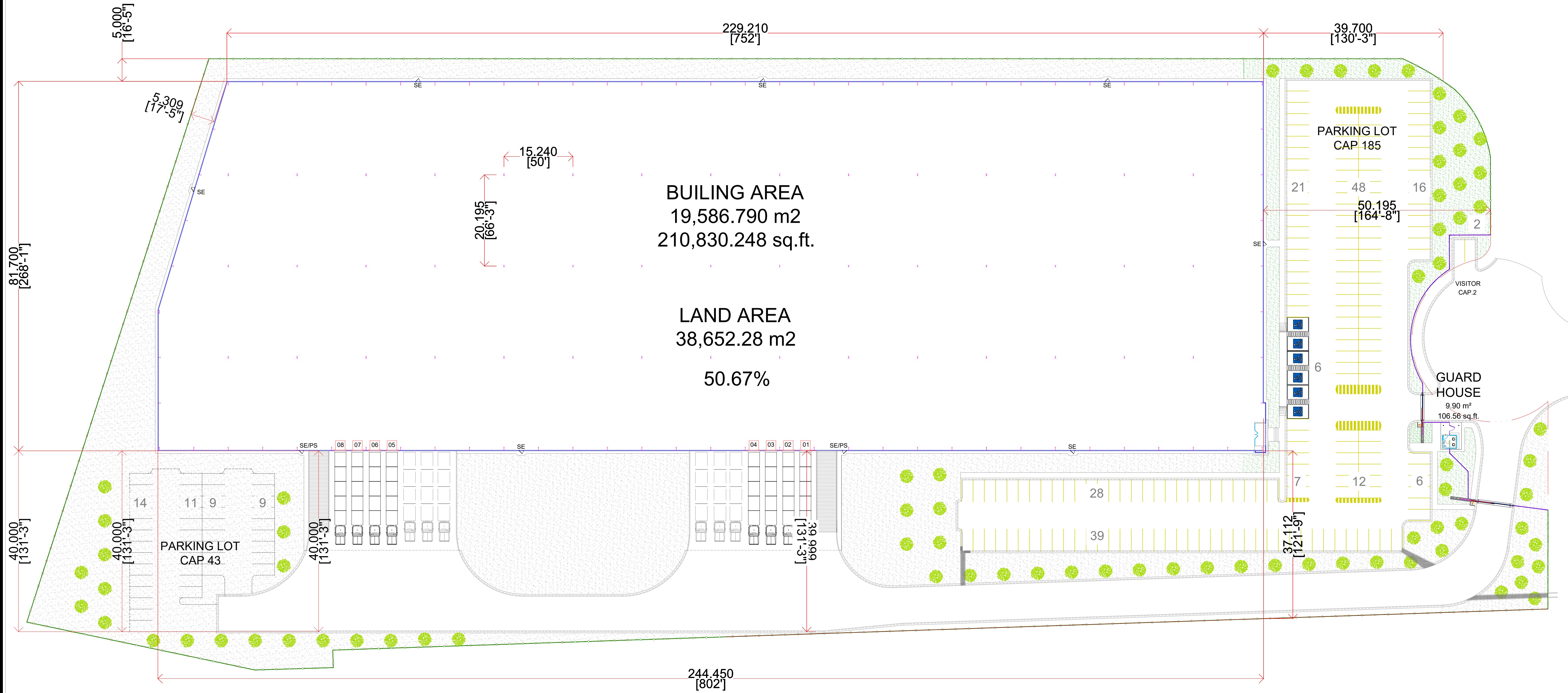
PLANTA ARQUITECTONICA ARCHITECTURAL LAYOUT
